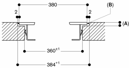
Longitudinal section
